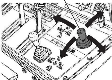
投雪方向調節レバー
