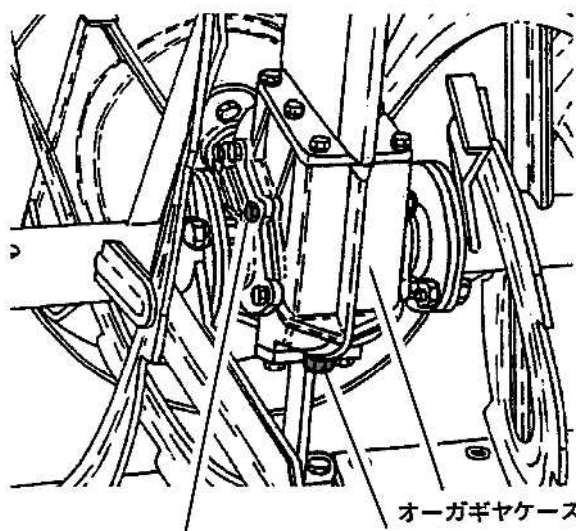
ドレンボルト
